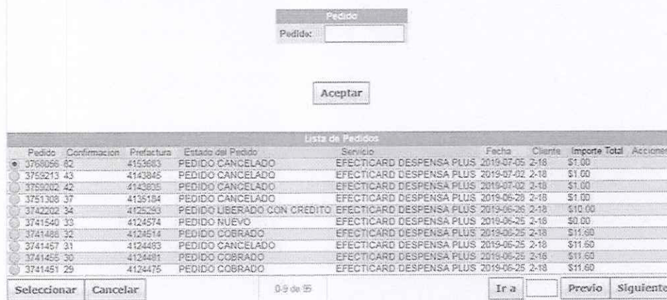
Figura 23. Pantalla Pedidos.
