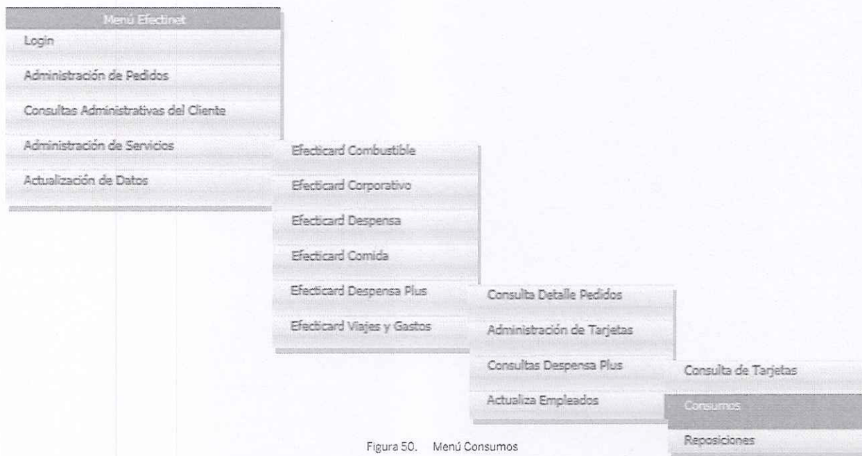
Figura 50. Menú Consumos
